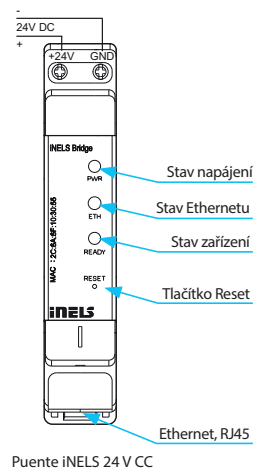
Puente iNELS 24 V CC
