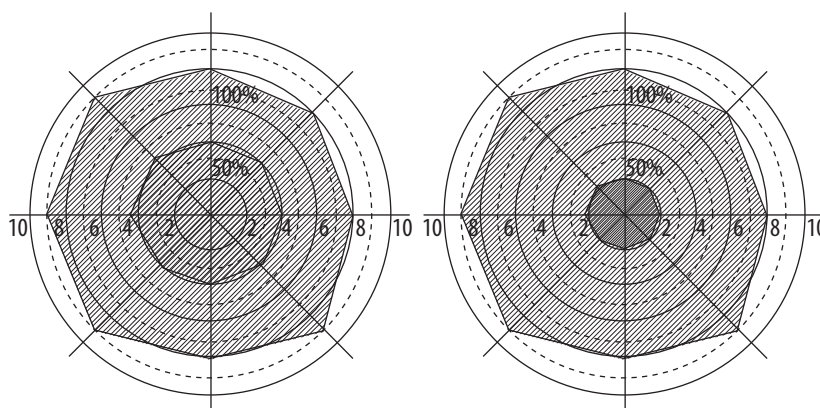
montážní výška stropu: 2,5 m nastavení rozsahu detekce: 100 % / 50 %
